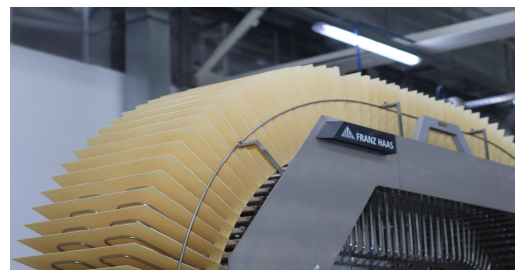
生产线
